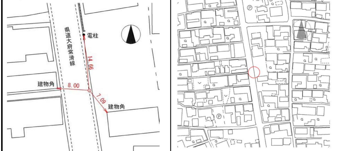
要図 縮尺: 1/500
