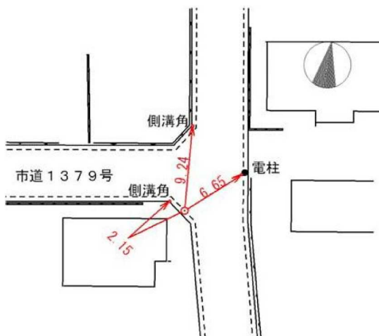
要図 縮尺: 1/500
