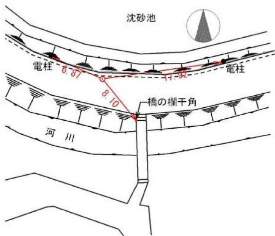
要図 縮尺: 1/500
