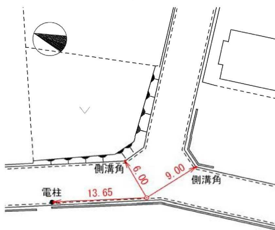
要図 縮尺: 1/500
