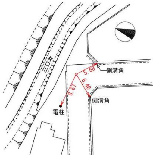
要図 縮尺: 1/500
