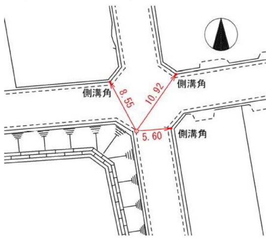
要図 縮尺: 1/500
