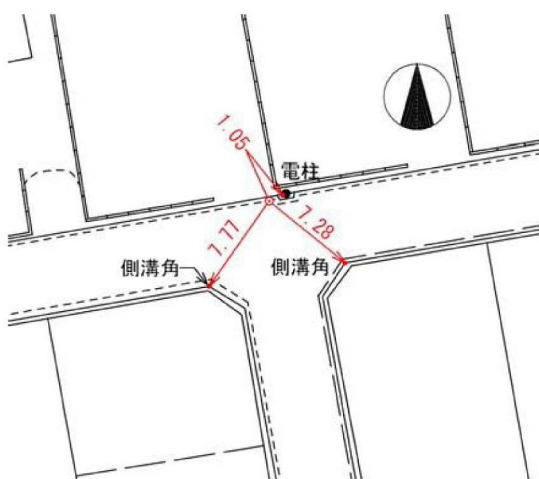
要図 縮尺: 1/500
