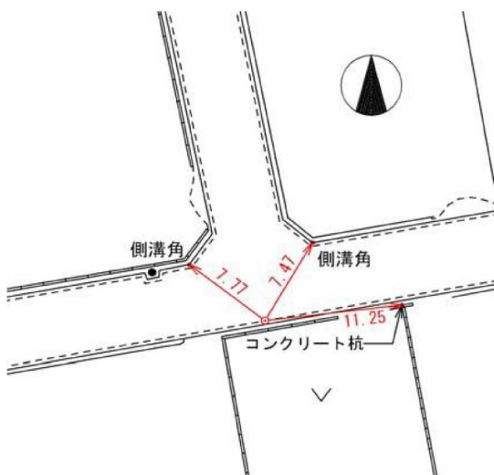
要図 縮尺: 1/500
