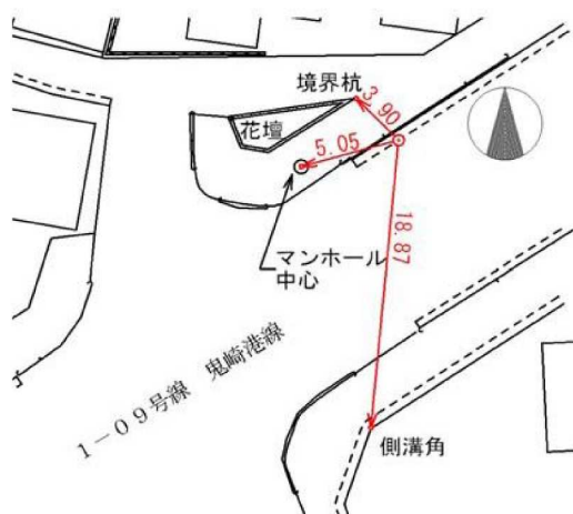
要図 縮尺: 1/500
