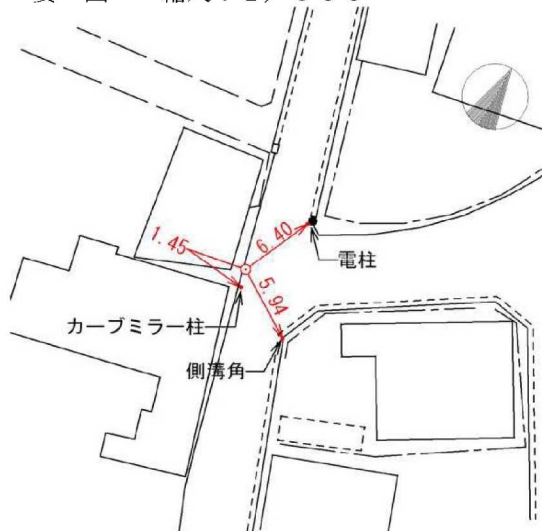
要図 縮尺: 1/500
